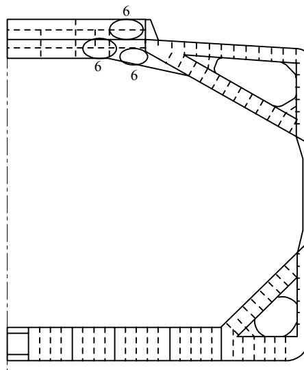
(d) Typical Hatch End Coaming Frame
